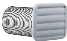
WEK 100, 120, 150 Wandeinbauset, flex. Rohr + Außenverschlussklappe. Bei WA Typen doppelter Verschluss. Wall mounting kit, flex. tube+pressure relief damper. For WA types double shutter.
