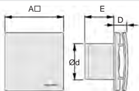
WEK 100, 120, 150 Wandeinbauset, flex. Rohr + Außenverschlussklappe. Bei WA Typen doppelter Verschluss. Wall mounting kit, flex. tube+pressure relief damper. For WA types double shutter.
